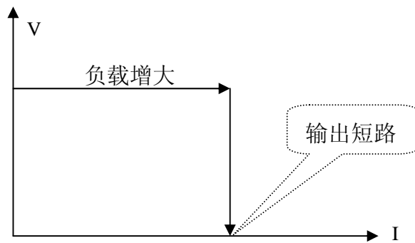
图 2： 整流模块输出特性
